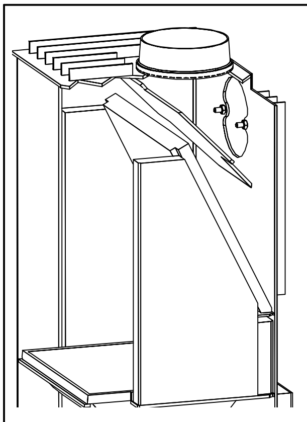
Lage des Feuerablenkvermiculit
