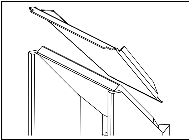
Lage des Feuerablenkrahmen
