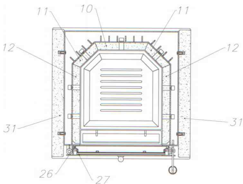
QUERSCHNITT VOM SCHARNIER DER FEUERRAUMTÜR
