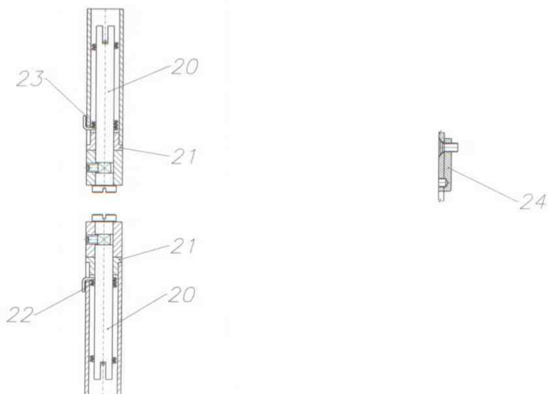
QUERSCHNITT VOM SCHARNIER DER FEUERRAUMTÜR
