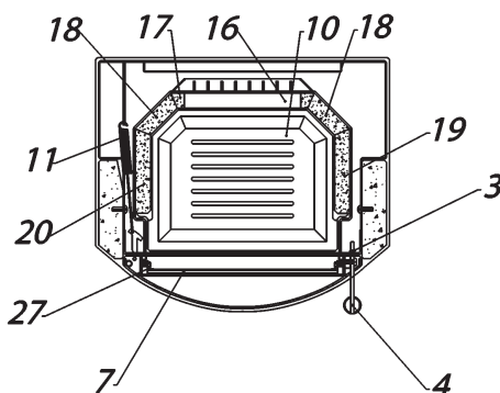
DETAILANSICHT
