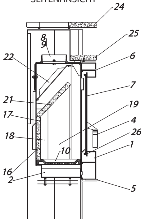
SEITENANSICHT
