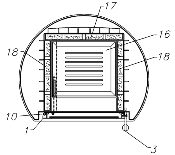
QUERSCHNITT VOM SCHARNIER DER FEUERRAUMTÜR
