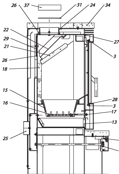
DETAILANSICHT
