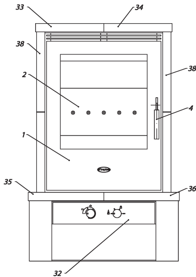
FRONTANSICHT
