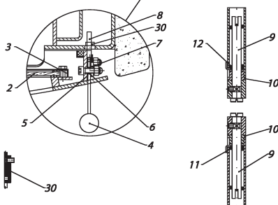
QUERSCHNITT VOM SCHARNIER DER FEUERRAUMTÜR
