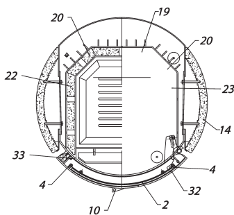
QUERSCHNITT VOM SCHARNIER DER FEUERRAUMTÜR
