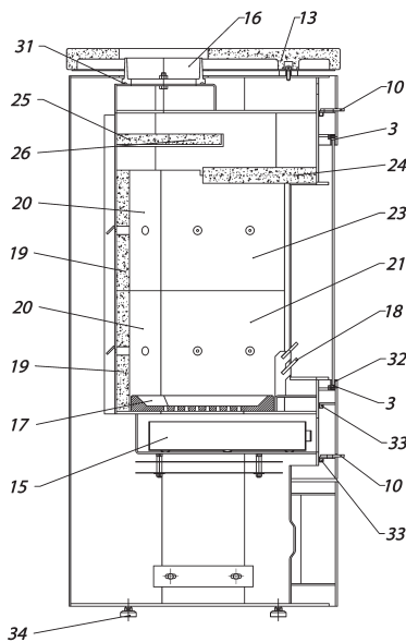
DETAILANSICHT
