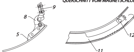
QUERSCHNITT VOM MAGNETSCHLOß
