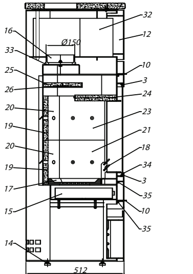
DETAILANSICHT
