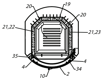
QUERSCHNITT VOM SCHLOßBLECH
