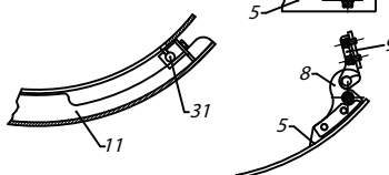
QUERSCHNITT VOM MAGNETSCHLOß
