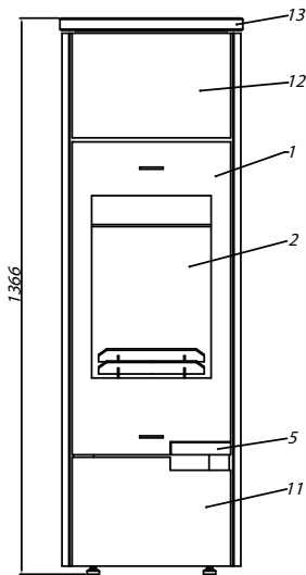
FRONTANSICHT
