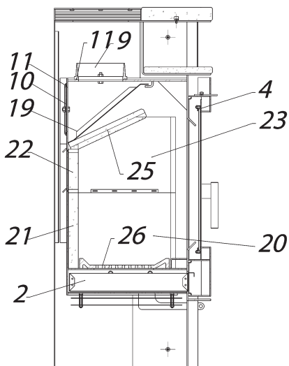
DETAILANSICHT
