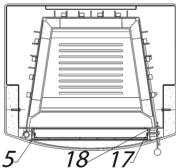
QUERSCHNITT VOM SCHARNIER DER FEUERRAUMTÜR
