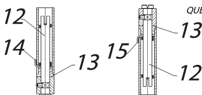
QUERSCHNITT VOM SCHARNIER DER FEUERRAUMTÜR
