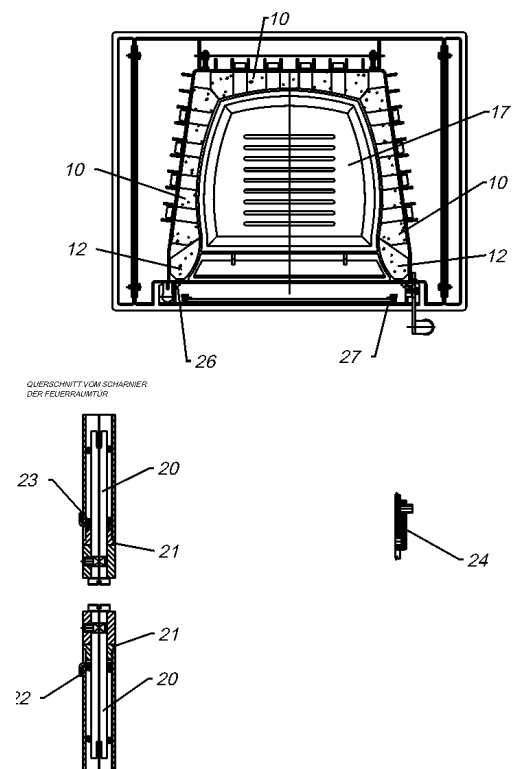
DETAILANSICHT
