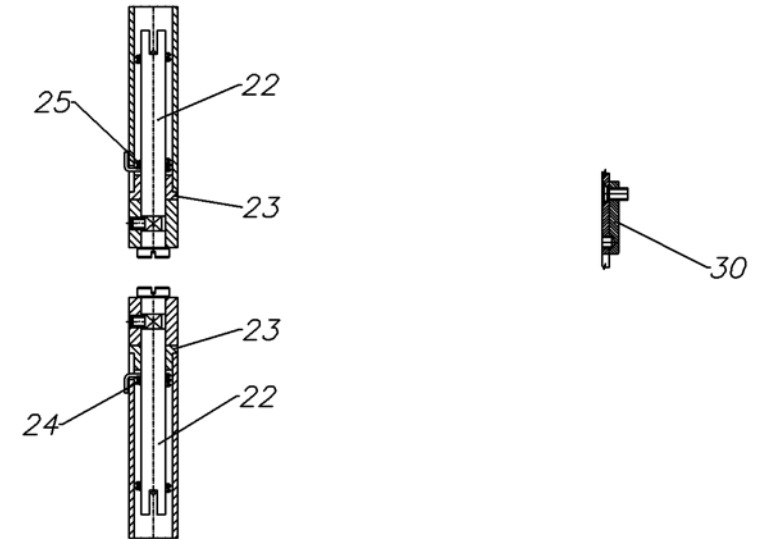
QUERSCHNITT VOM SCHARNIER DER FEUERRAUMTÜR
