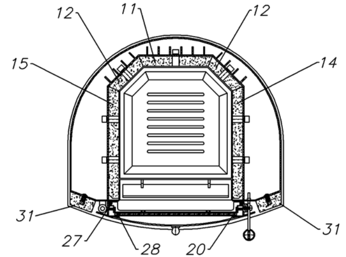
QUERSCHNITT VOM SCHARNIER DER FEUERRAUMTÜR
