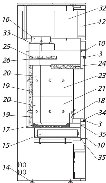
DETAILANSICHT
