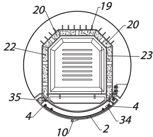
QUERSCHNITT VOM MAGNETSCHLOß
