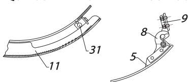
QUERSCHNITT VOM SCHARNIER DER FEUERRAUMTÜR
