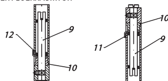
QUERSCHNITT VOM SCHARNIER DER FEUERRAUMTÜR
