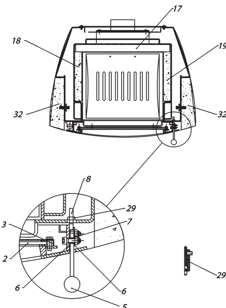
DETAILANSICHT
