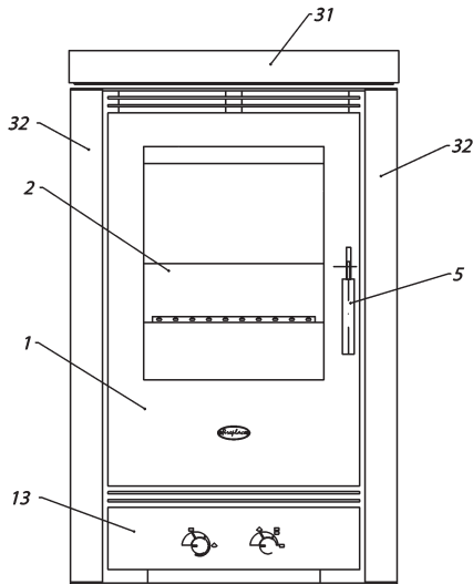
FRONTANSICHT
