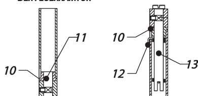
QUERSCHNITT VOM SCHARNIER DER FEUERRAMTÜR
