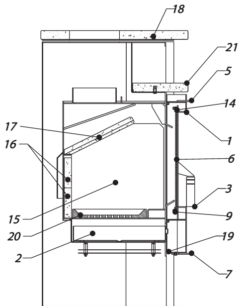
SEITENANSICHT
