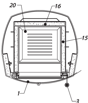
QUERSCHNITT DES SCHLOßBLECHS
