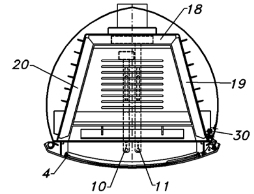
QUERSCHNITT VOM SCHLOBBLECH
