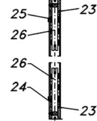
QUERSCHNITT VOM SCHARNIER DER FEUERRAUMTÜR
