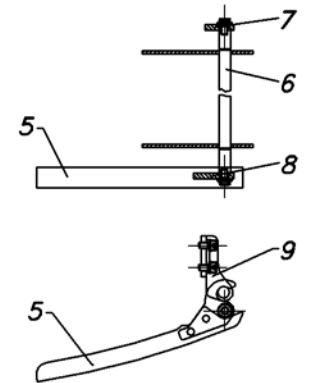
QUERSCHNITT VOM SCHLOBBLECH
