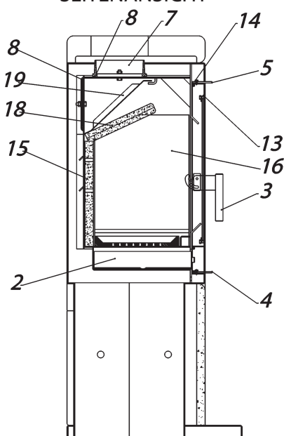
SEITENANSICHT
