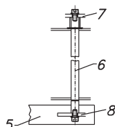
QUERSCHNITT VOM SCHLOBBLECH
