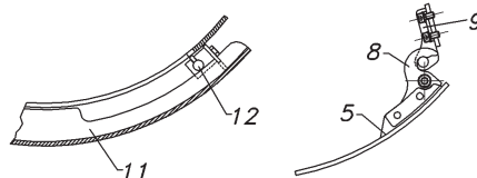
QUERSCHNITT VOM MAGNETSCHLOß
