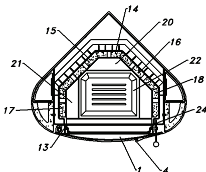
QUERSCHNITT VOM SCHARNIER DER FEUERRAUMTÜR
