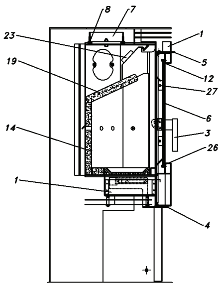
SEITENANSICHT
