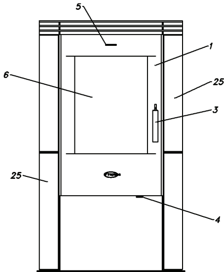
FRONTANSICHT
